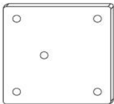
MLCAL38-4.7 冲孔铝配件SIZE: 2"X3"X3/16 H: 1-5/8" 380/box
